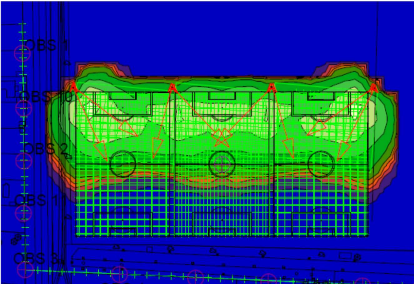
Figurer; Placering af armaturer og master i områder. Nye armaturer på halvbanerne 5,8,11 omfatter denne ansøgning. Beregningerne viser et meget lavt lysspild udenfor halvbanerne.
