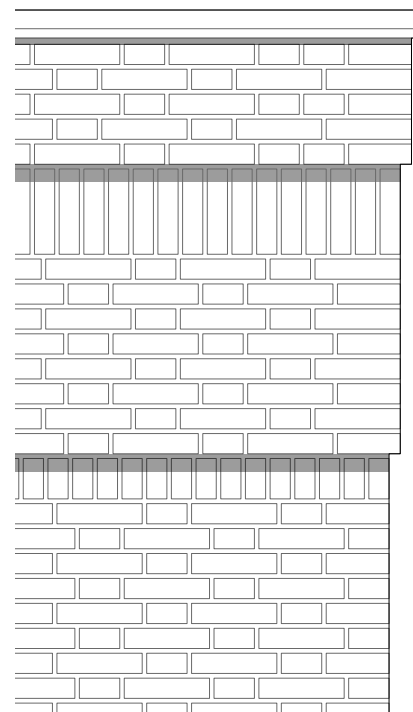
Principtegning af murkrones gesims på det nord-østlige hjørne mod Nordre Fasanvej
