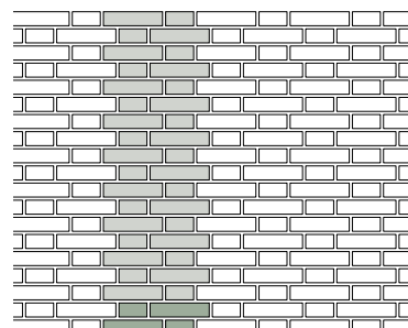
Detaljer i facaden udvalgte steder: Et levende spil mellem kopper og løbere i et engelsk forbandt giver de forholdsvis store murede flader en dekorativ virkning på afstand.
